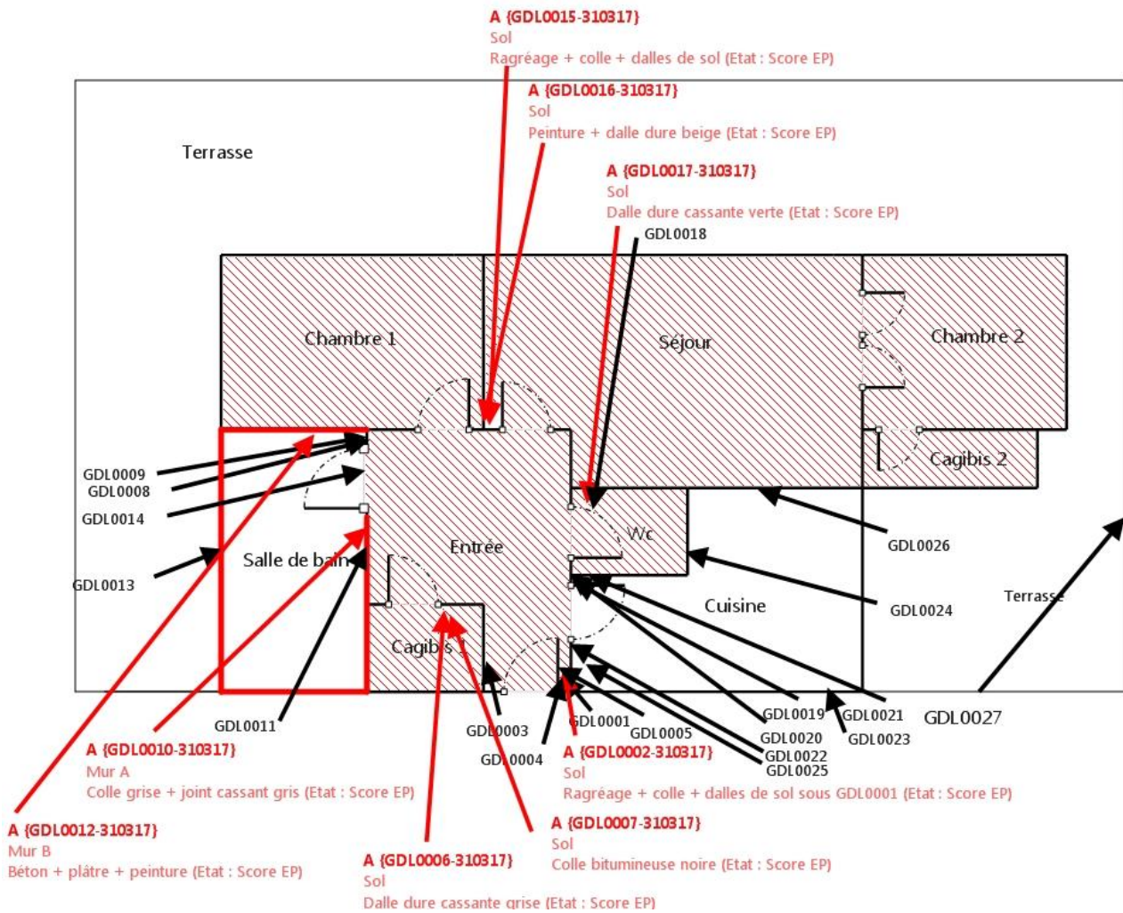
Planche (croquis) de repérage technique effectué par le cabinet : ALLODIAGNOSTIC, auteur : Geraud DE LAFFON Dossier n° 862733 du Adresse du bien : 4 SQUARE PAUL ALGIS ESC AD 50LAD0603 (50LAD0603) 77360 VAIRES SUR MARNE
